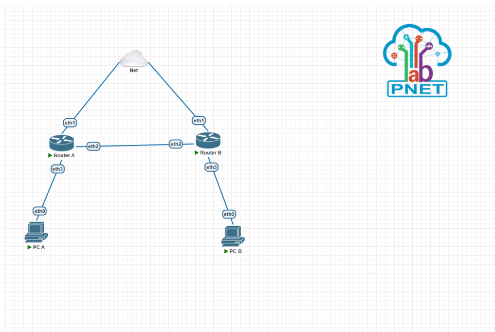
Gambar 2: Topologi jaringan pada PNET Lab
